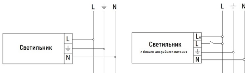
Рис. 2. Схемы подключения к сети
