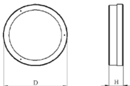
Рис. 1. Общий вид светильника
