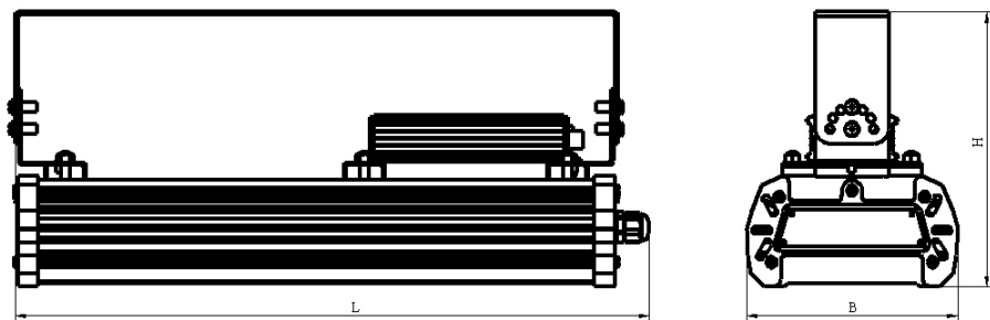
Рис. 1. Общий вид светильника
